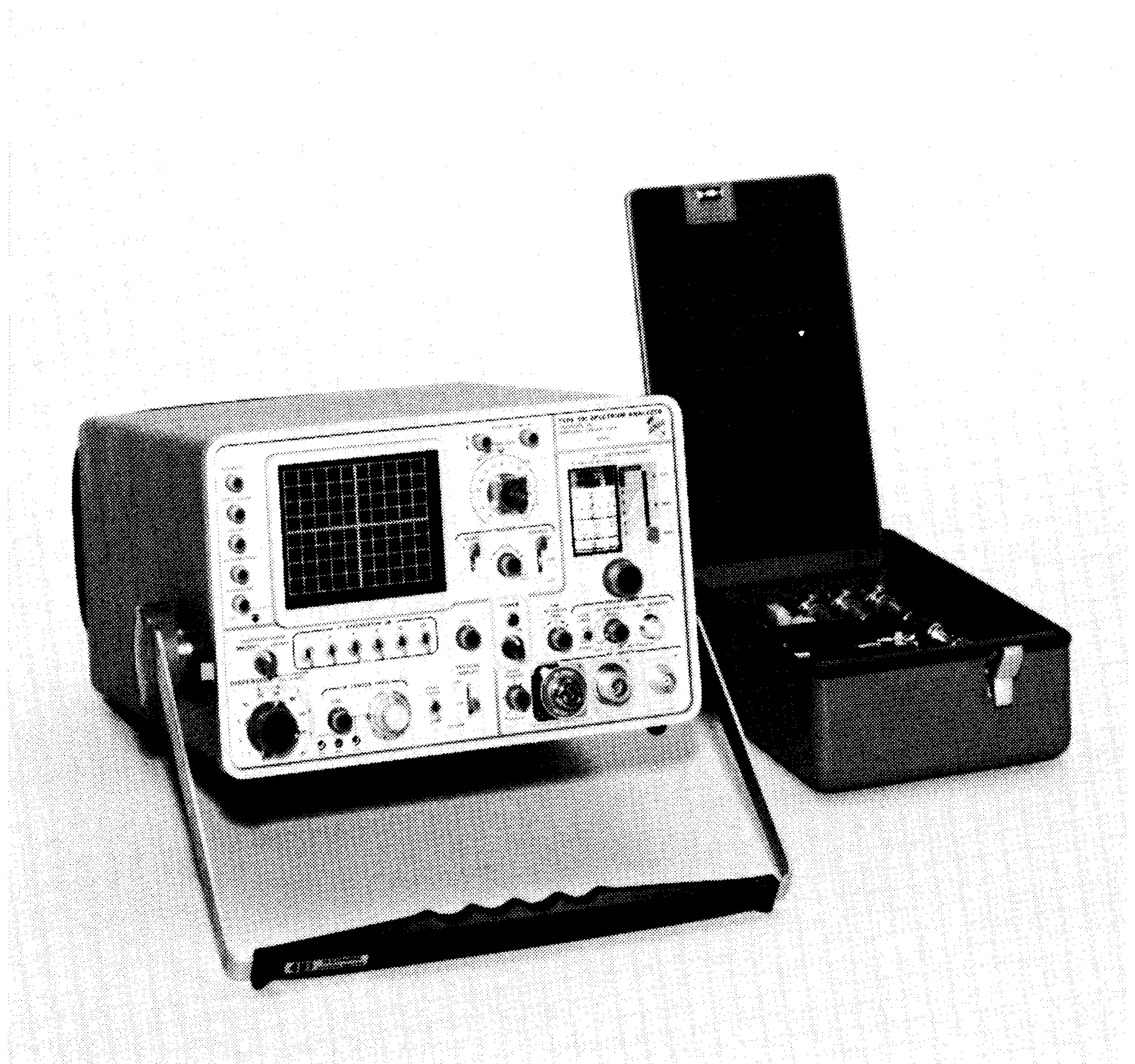
Fig. 1-3. Tektronix Type 491.
